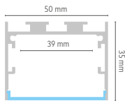
Perfil SPACE 50mm de superficie.
