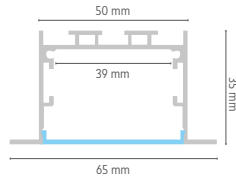
Perfil SPACE 50mm empotrable.
